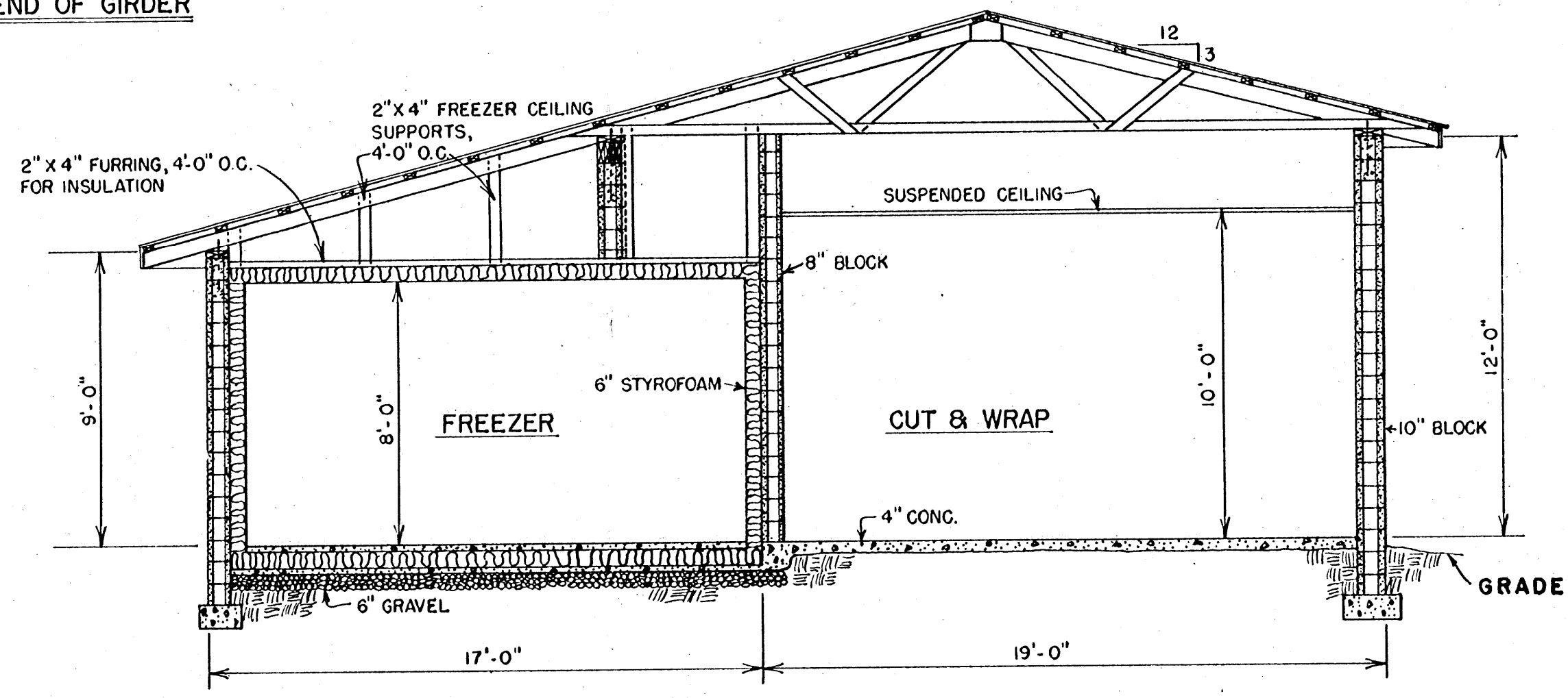
SECTION C-C SCALE: 1/4" = 1'-0" 12'-0" 1' 2' 3"
