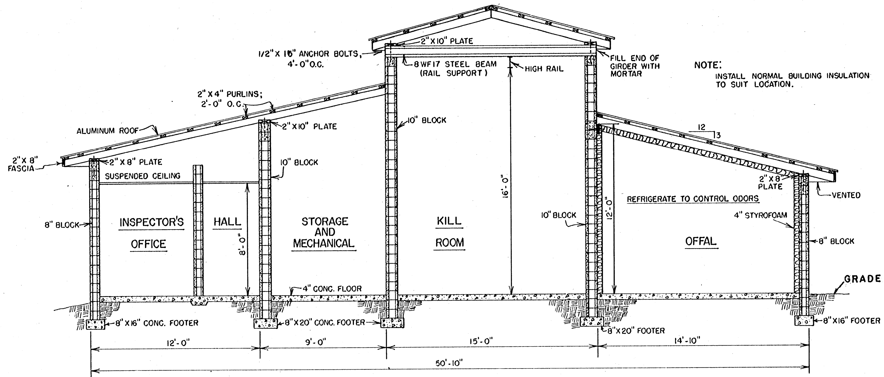
SECTION A-A SCALE: 1/4"=1'-0"
